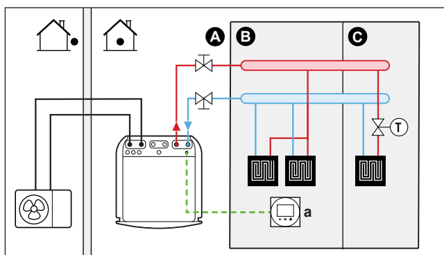
A Hovedafgangsvandtemperaturzone
