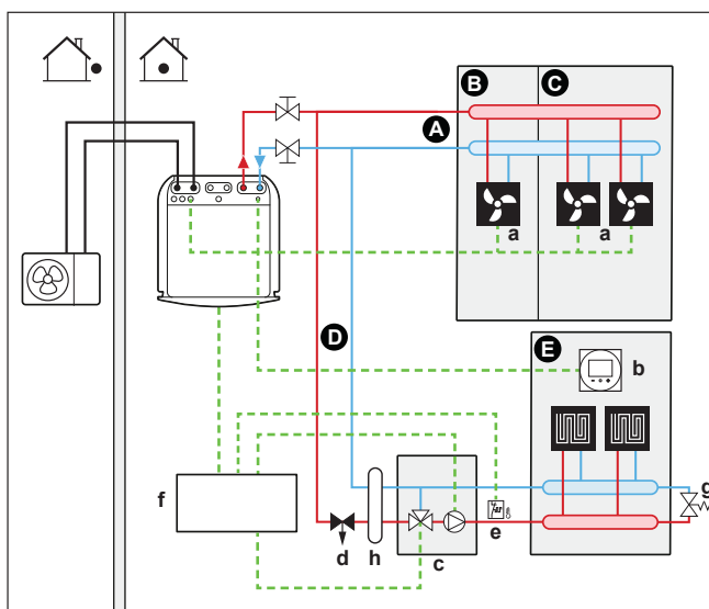
3 System med hydraulisk udskiller til begge zoner: Til dette system kræves en direkte pumpe til den ekstra zone.
