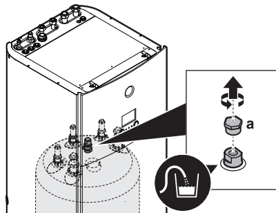
a Adgangspunkt til tank
