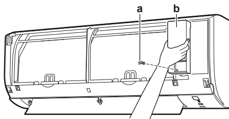
a Skruer til servicedæksel b Servicedæksel
