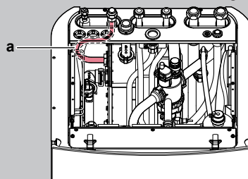
a Kølemiddelløbet
