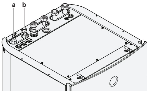
a Tilslutning for flydende kølemiddel b Tilslutning for kølegas
